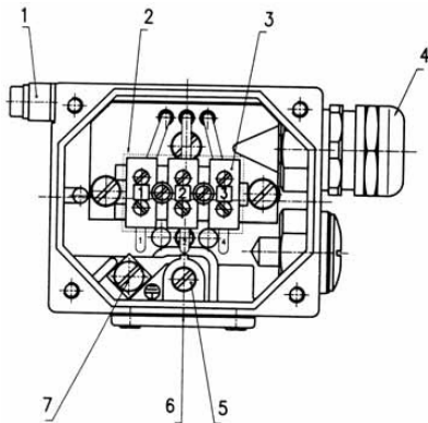
Fig. 21. Schaltpunkteinstellung
